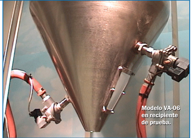
Modelo VA-06 (con válvula solenoide, acoplamiento de montaje y tuerca de fijación)
